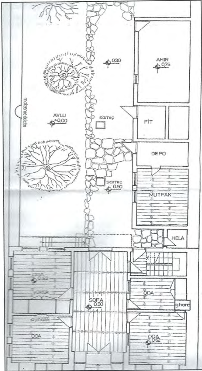
Şekil 3.12. Ada: 347, Parsel: 2, Tescil No:9, Osman Öz Evi'nin zemin katındaki müştemilatında 'fit' mekanının konumu (Yapının planı: Çetin, 2000).
