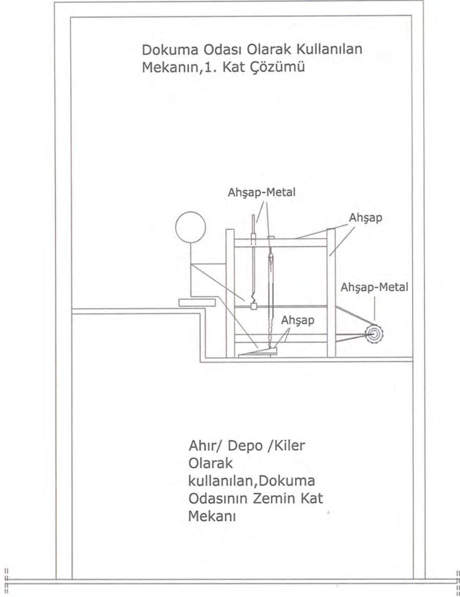
Şekil 3.11. Dokuma odası olarak kullanılan mekanın, 1. kat çözümü (Seda Şimşek Tolacı çizim ve fotoğraf arşivi, 2005-2009)
