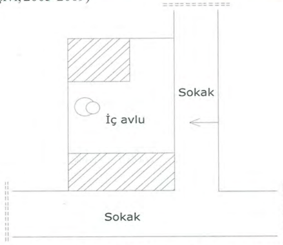
Şekil 3.94. Burdur Türk Evi'ndeki kamusal alan -özel alan ilişkisinde 6.tip (Seda Şimşek Tolacı çizim ve fotoğraf arşivi, 2005-2009)
