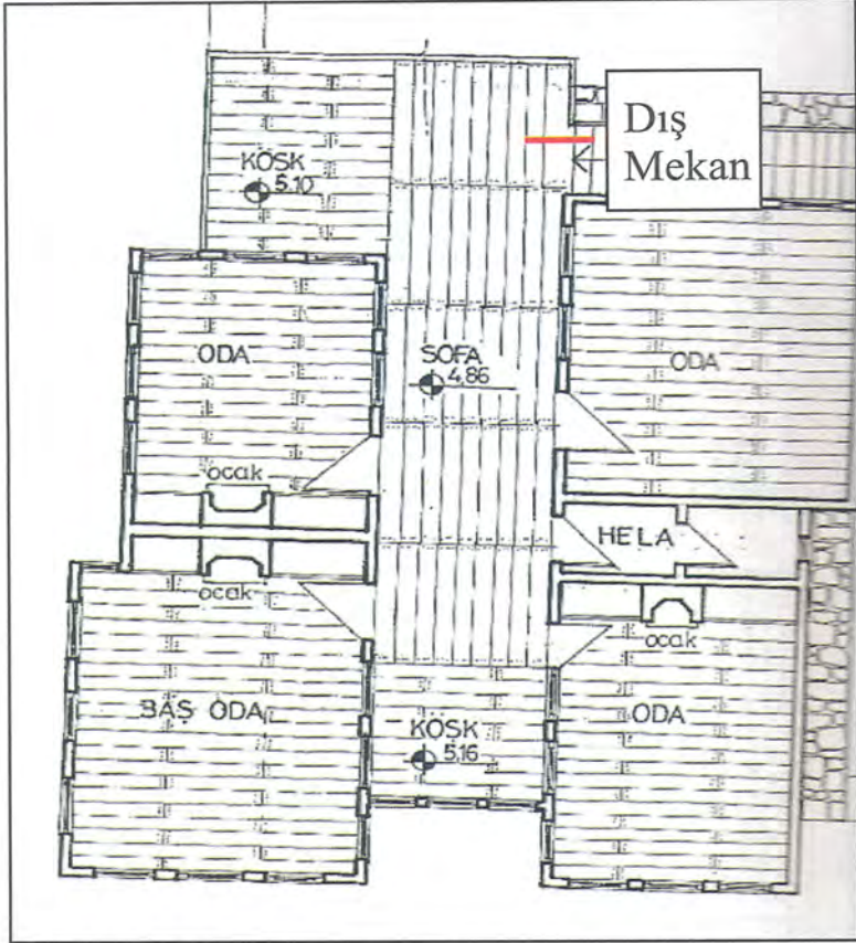
Şekil 3.58. Mısırlılar Evi birinci kat planı (Çetin İğci, 2000)
