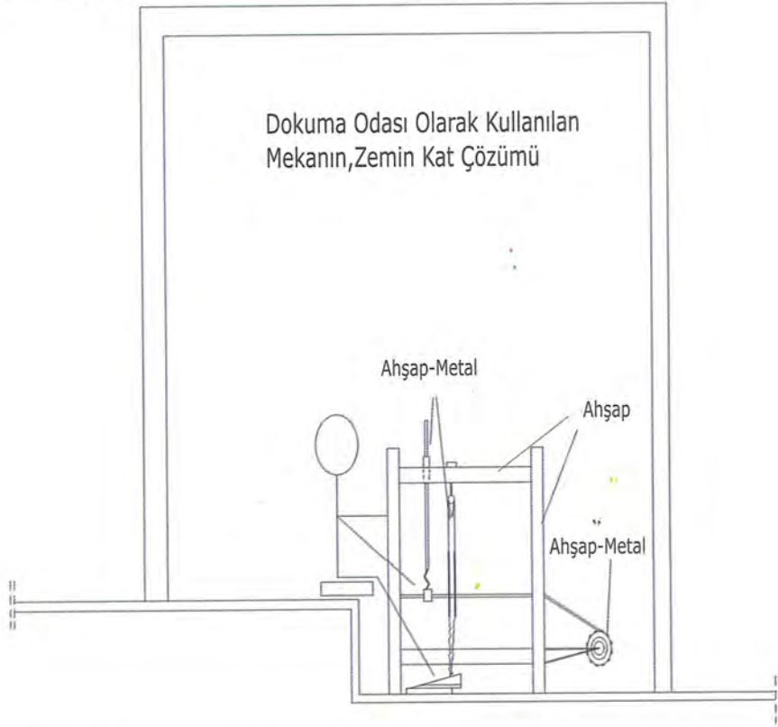
Şekil 3.10. Dokuma odası olarak kullanılan mekanın, zemin kat çözümü(Seda Şimşek Tolacı çizim ve fotoğraf arşivi, 2005-2009)
