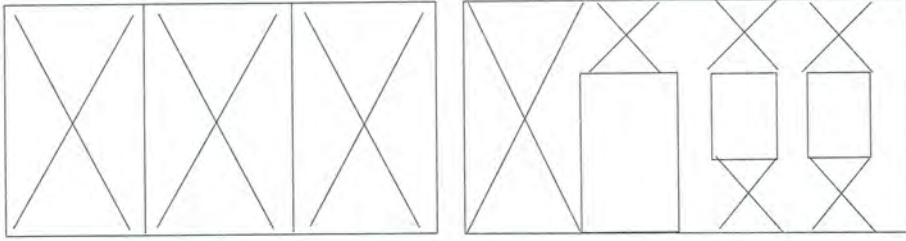
Şekil 3.154. Ahşap karkasın, sağır cephe ve açıklıkları olan cephede uygulanış şeması (Seda Şimşek Tolacı çizim ve fotoğraf arşivi, 2005-2009)
