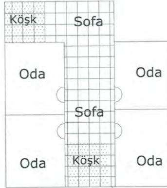
Şekil 4.6. İncelenen Türk Evlerinde, tek sofanın açık ve kapalı mekana sahip olduğu plan tipi (Seda Şimşek Tolacı çizim ve fotoğraf arşivi, 2005-2009)
