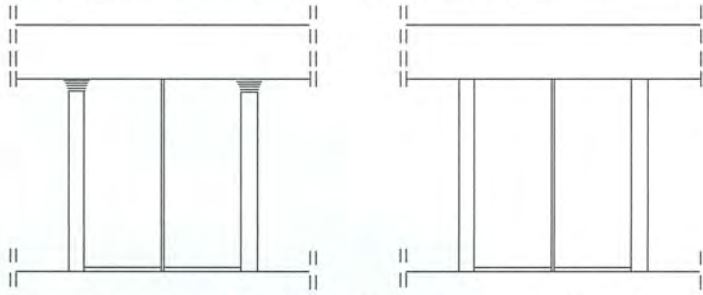
Şekil 2.29. Tarihi Ticari Merkez'de kemersiz cephe biçimlenişleri (Seda Şimşek Tolacı çizim ve fotoğraf arşivi, 2005-2009)
