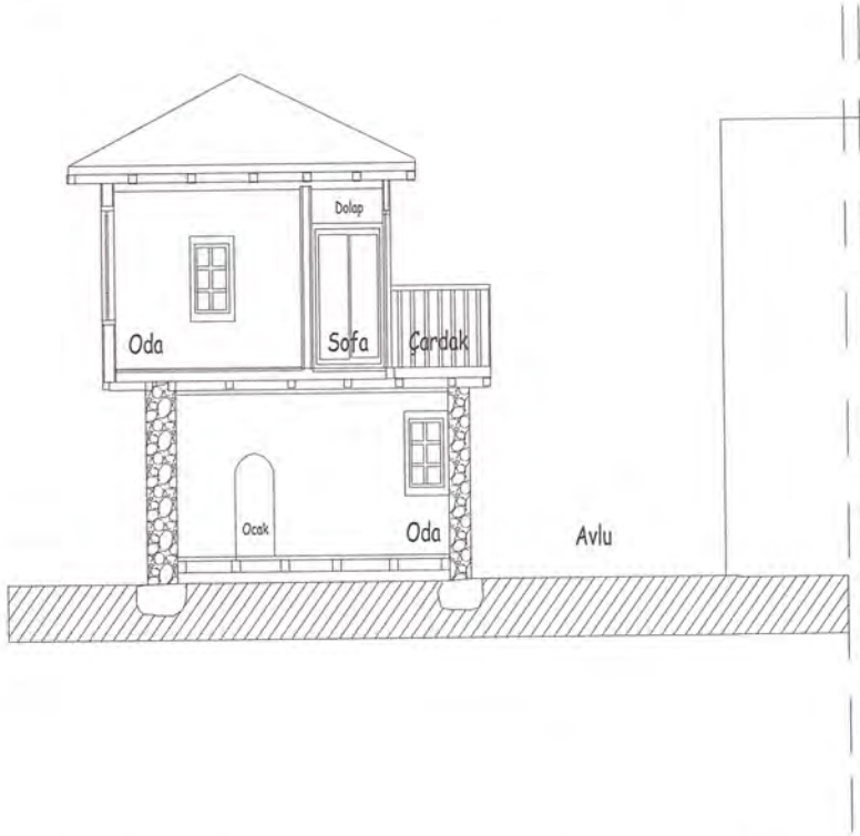
Şekil 3.21. Osman Uysal Evi'nde çardak -yapı- avlu ilişkisi (Seda Şimşek Tolacı çizim ve fotoğraf arşivi, 2005-2009)
