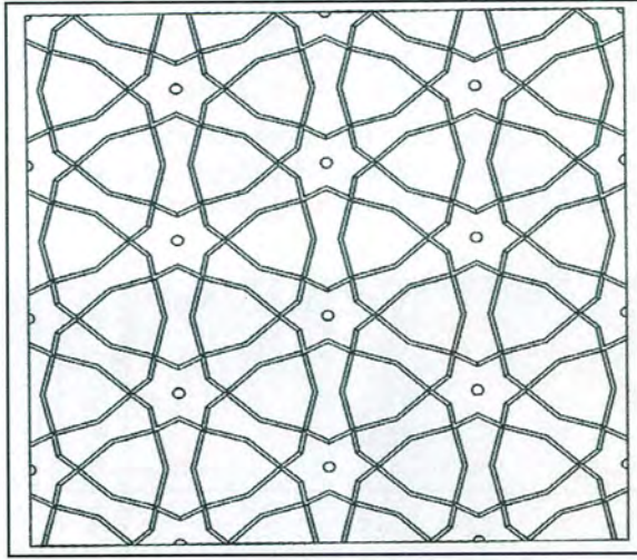
Şekil 3.141. Bakibey Konağı, başoda, seki üstü tavan detayı (Şimşek ve Önkol, 2006)
