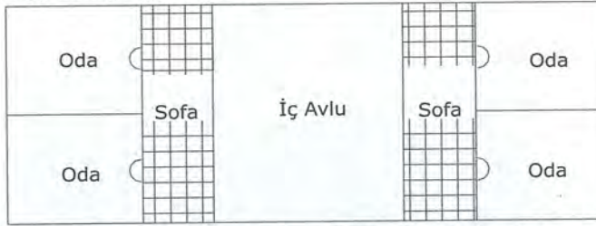
Şekil 3.49. Burdur Türk Evi iç avlulu, çift yapılı evlerin plan şeması (Osman Uysal Evi ve Yağcı Kadirler Evi) (Seda Şimşek Tolacı çizim ve fotoğraf arşivi, 2005-2009)
