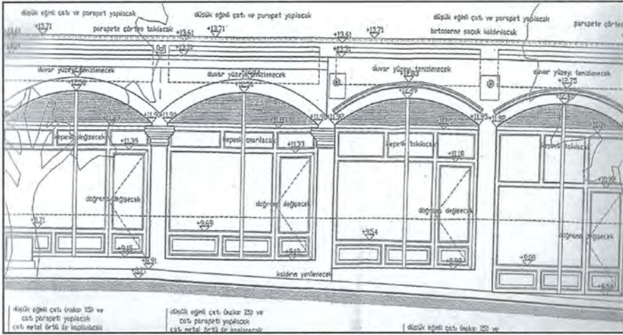
Şekil 2.22. Tarihi Ticari Merkez'de, eğime paralel olarak gelişen 1. Yağ Pazarı Sokak üzerindeki ticari yapıların konumlanması -Adres Adres:Ulu Cami ve Saat Kulesi Mevkii,1. Yağ Pazarı Sokak No:2-4-6-8 (Yapıya ait cephe çizimi, Uslular İnşaat Proje, Restorasyon L.t.D. Ş.T.İ.'den temin edilmiştir.
