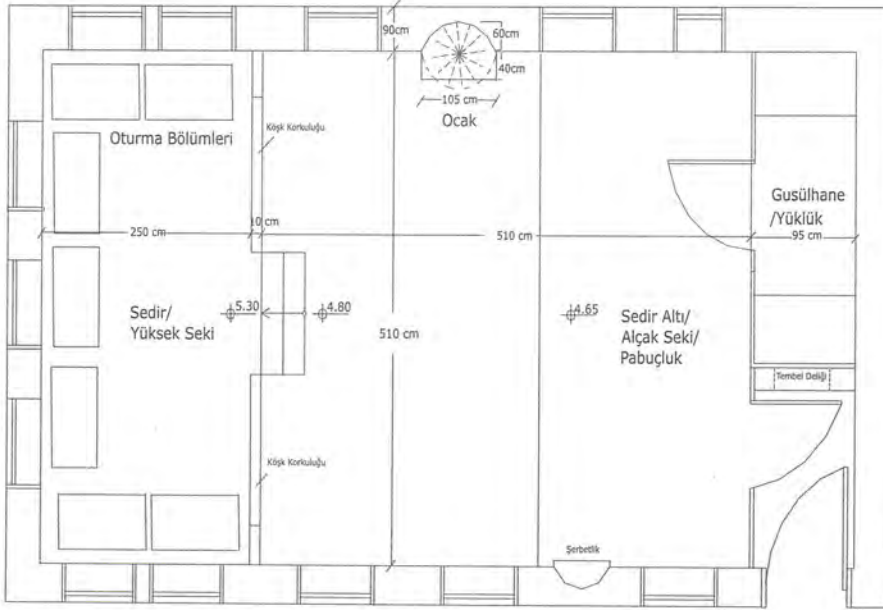
Şekil 3.72. Baki Bey Konağı baş odasının planı (Seda Şimşek Tolacı çizim ve fotoğraf arşivi, 2005-2009)
