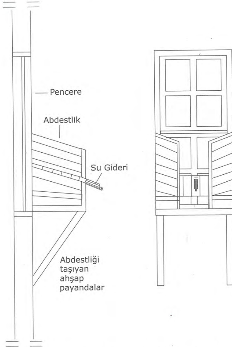
Şekil 3.69. İç sofanın dışa açılım yaptığı yerde, dış mekana taşırılarak yapılan tezgah şeklindeki abdestliğin kesit ve görünüşü (Seda Şimşek Tolacı çizim ve fotoğraf arşivi, 2005-2009)
