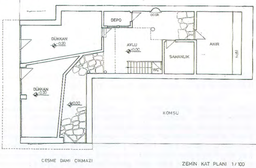
Şekil 3.95. Yapı tescil numarası 40 olan Yağcı Kadirler Evi'nin zemin kat planı (Çetin, 2000)
