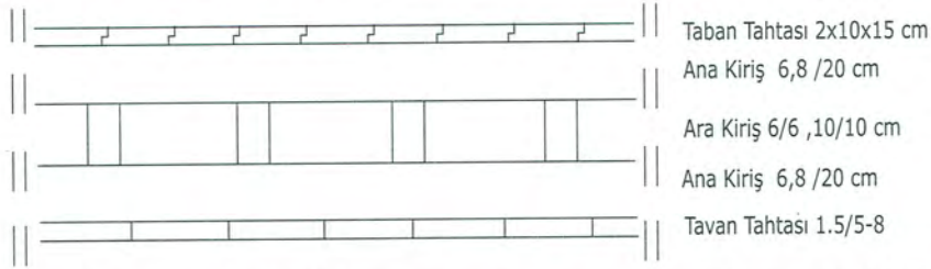
Şekil 3.159. Burdur Türk Evlerinde kullanılan döşemelerin kesiti(Seda Şimşek Tolacı çizim ve fotoğraf arşivi, 2005-2009)
