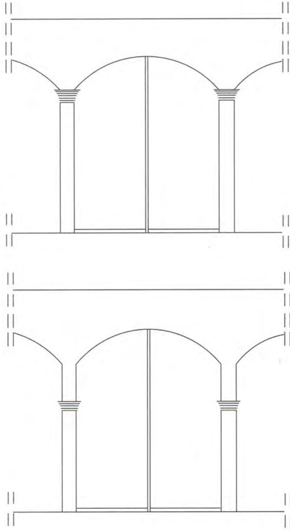
Şekil 2.26. Tarihi ticari merkezde hakim olan basık kemerli cephe tipinde, sütun başlıklarının yerleri (Seda Şimşek Tolacı çizim ve fotoğraf arşivi, 2005-2009)
