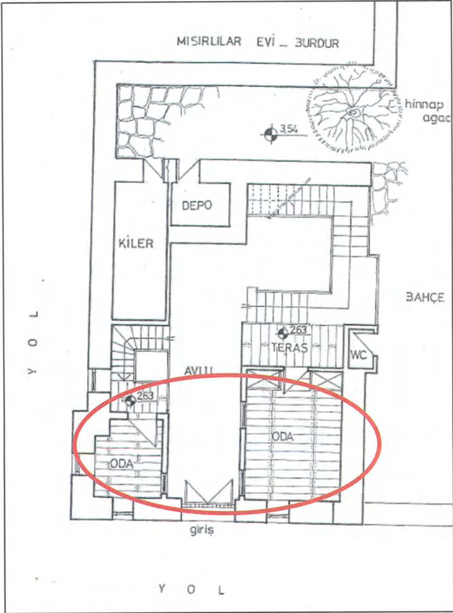
Şekil 3.57. Mısırlılar Evi'nin ara kat planı (Çetin, 2000)
