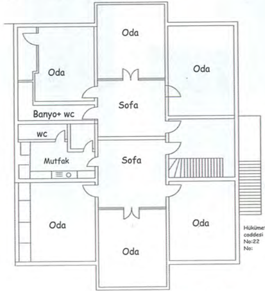
Şekil 3.46 Orta sofalı plan tipi mekan örgütlenmesi şeması (Seda Şimşek Tolacı çizim ve fotoğraf arşivi, 2005-2009)
