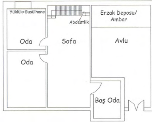
Şekil 3.37. Tescil numarası 1 olan yapının sofa- mekan ilişkisi (Seda Şimşek Tolacı çizim ve fotoğraf arşivi, 2005-2009)
